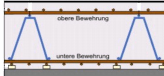
Sichtbetonabstandhalter
